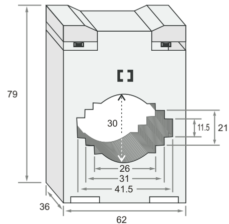
Outer Dimension: 62 x (W) x 79 (H) x 36 (D)
